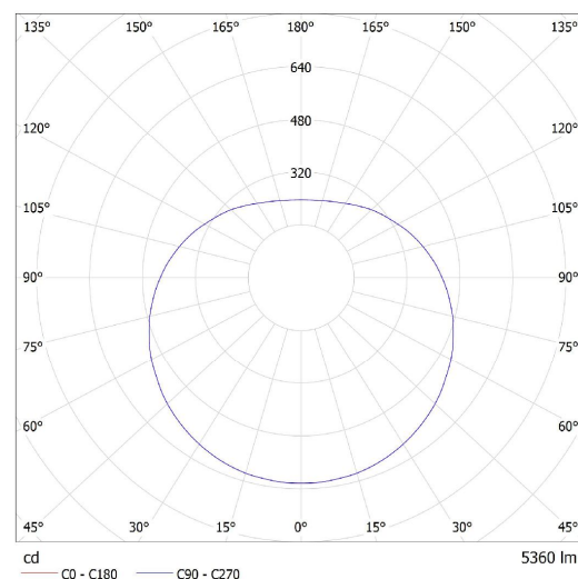
Lucis ZL1.PX4.400 PE DIADEM PE LED / LDC (Polar)
